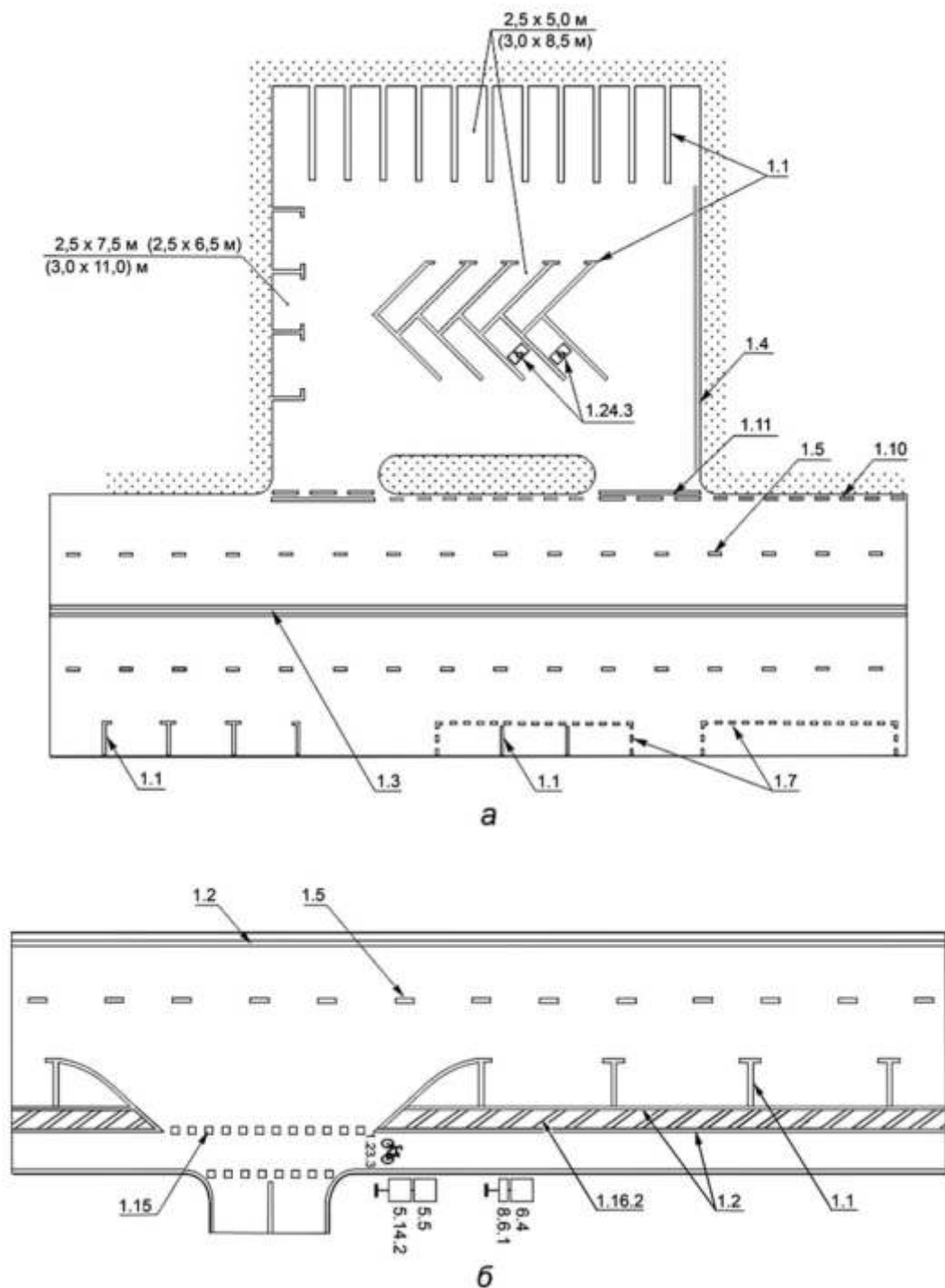
а - пример нанесения разметки в местах организованной парковки транспортных средств на проезжей части и прилегающей территории; б - пример нанесения разметки в местах организованной парковки транспортных средств с устройством велополосы
