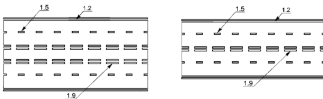
Рисунок В.17 - Примеры нанесения разметки 1.9
