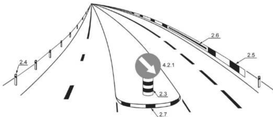
Рисунок В.24 - Пример нанесения разметки 2.3 - 2.7
