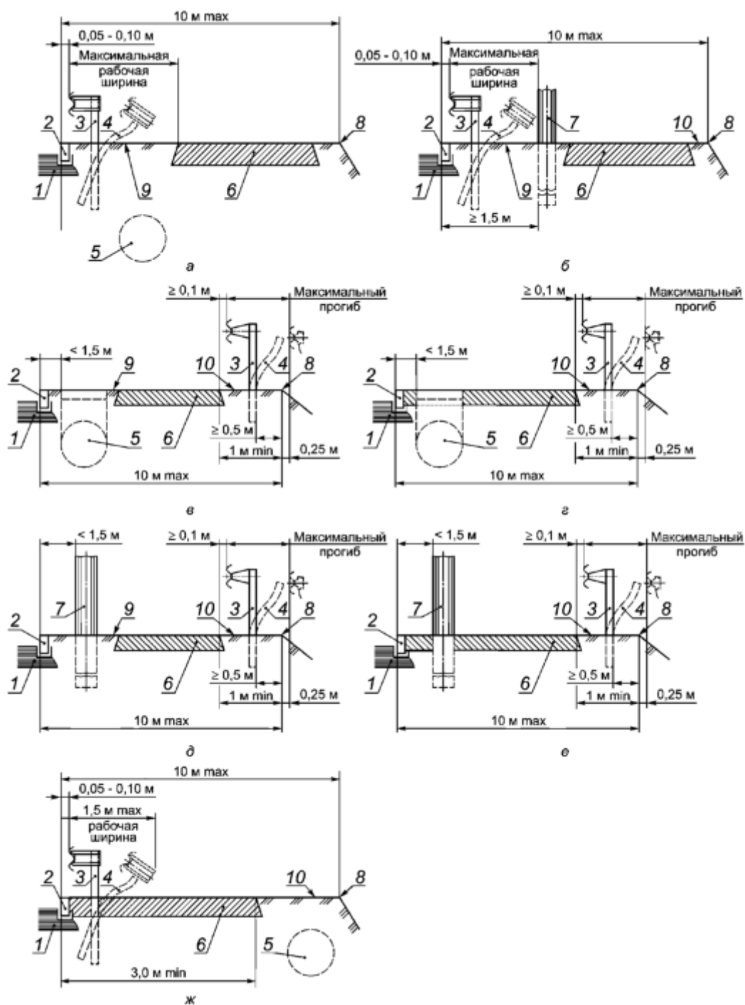
Рисунок В.28 - Примеры установки дорожных ограждений
