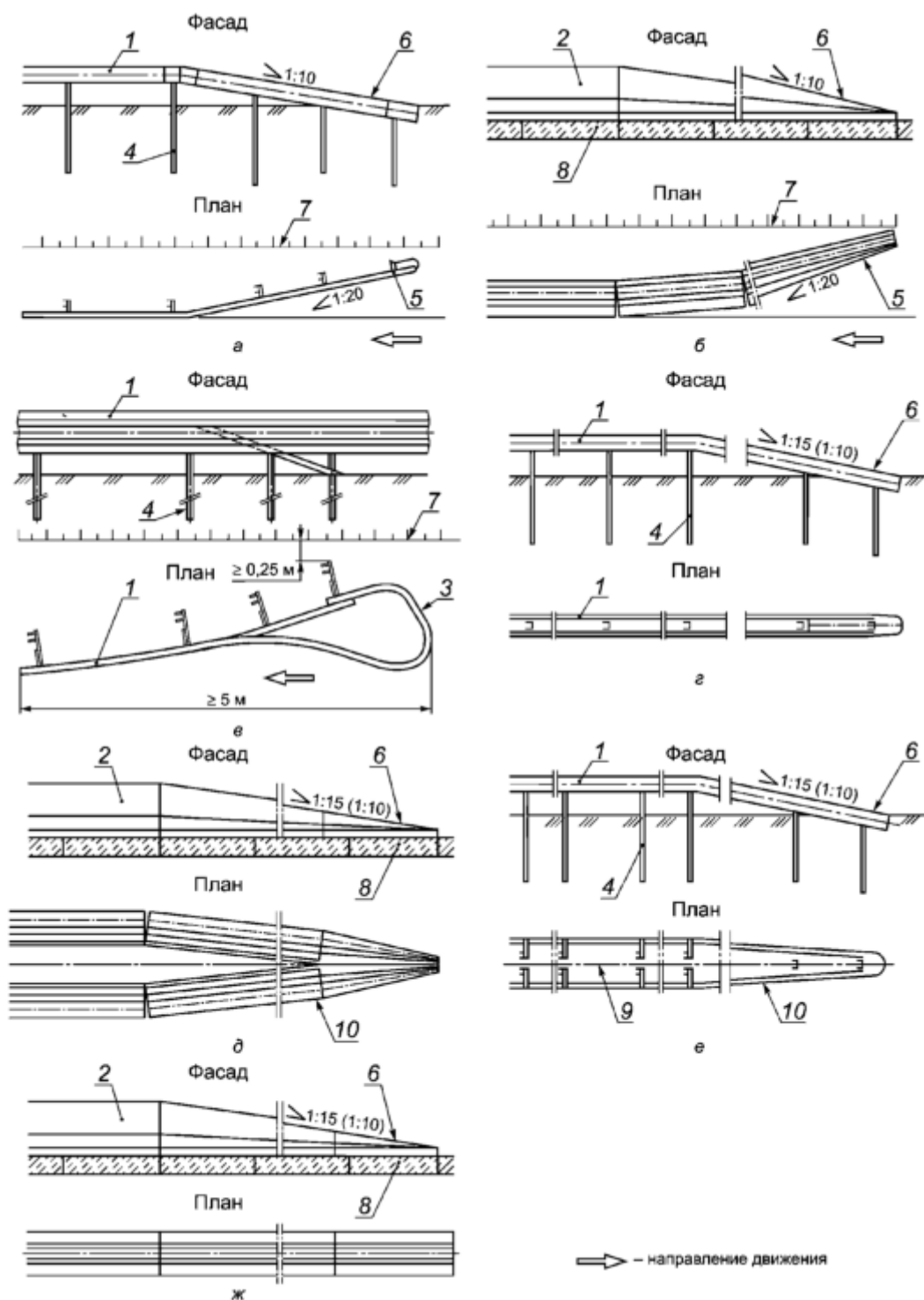
Рисунок В.29 - Примеры установки дорожных ограждений
