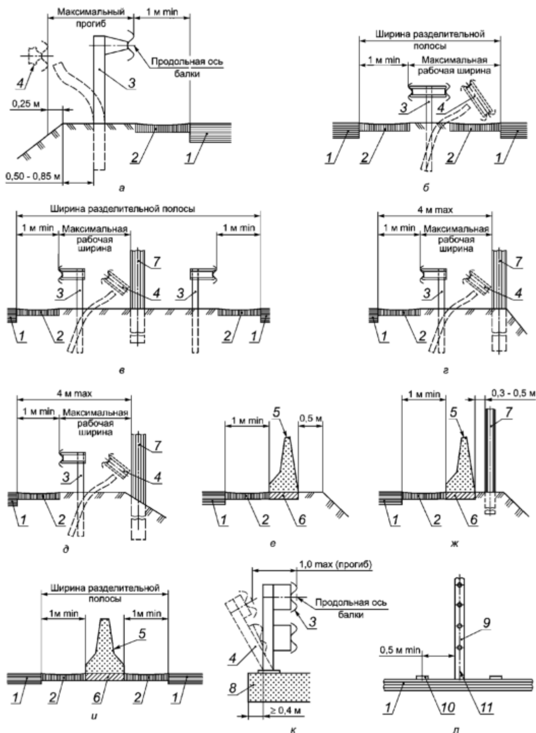
Рисунок В.27 - Смещение дорожного ограждения
