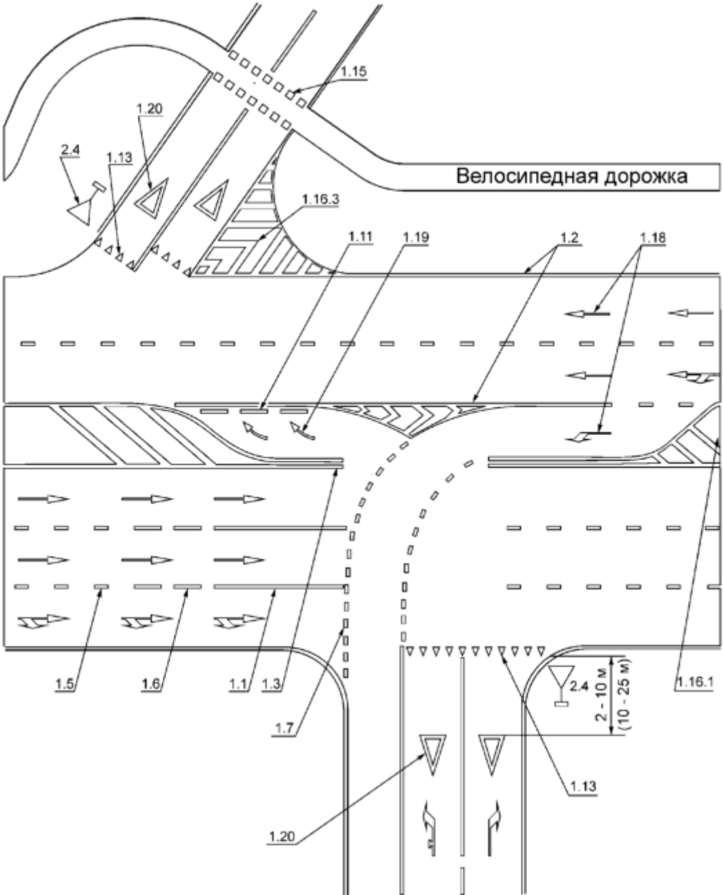
Рисунок В.10 - Пример нанесения разметки канализированного пересечения
