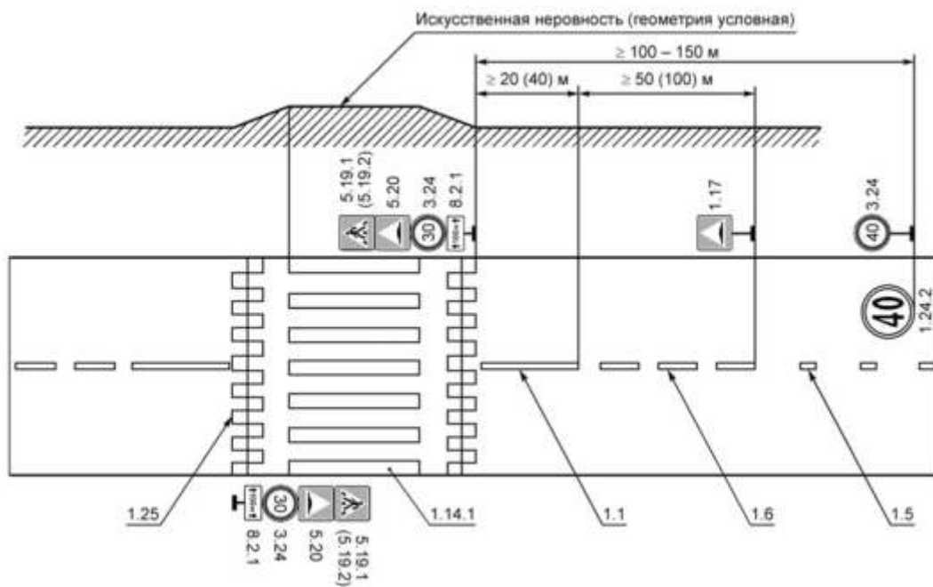
Рисунок В.21 - Пример нанесения разметки 1.25
