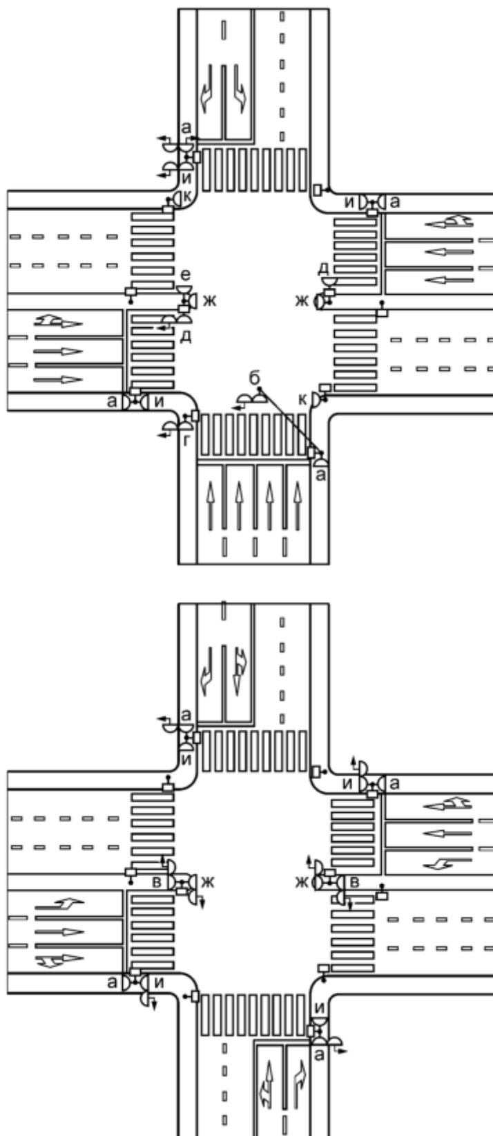
а - к - места установки светофоров по 7.4.1
